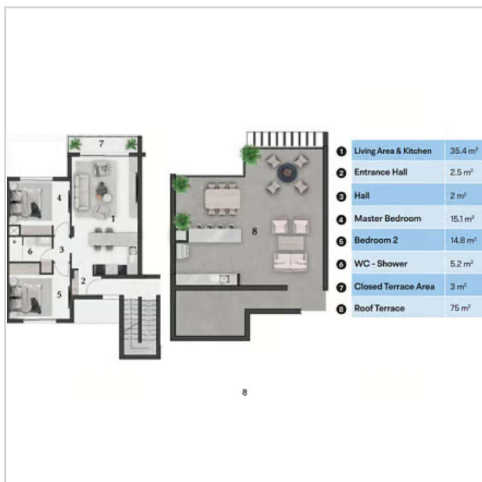
3-ZKB-Penthouse Grundriss
